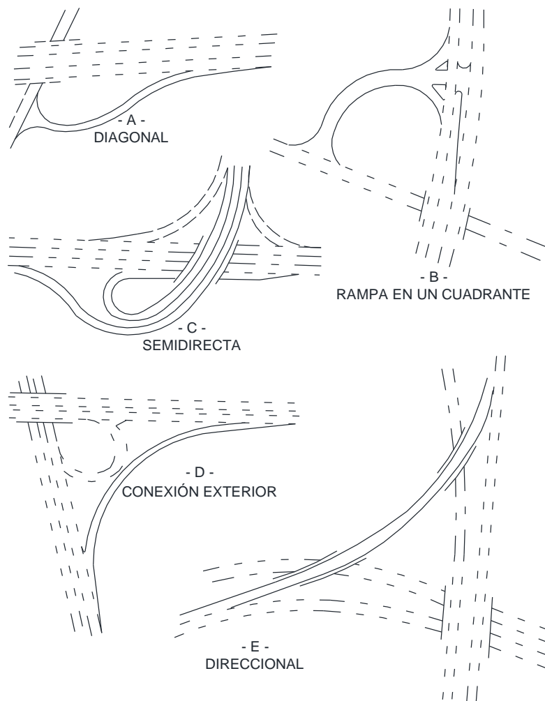
FIGURA IX.27. Tipos generales de enlaces
