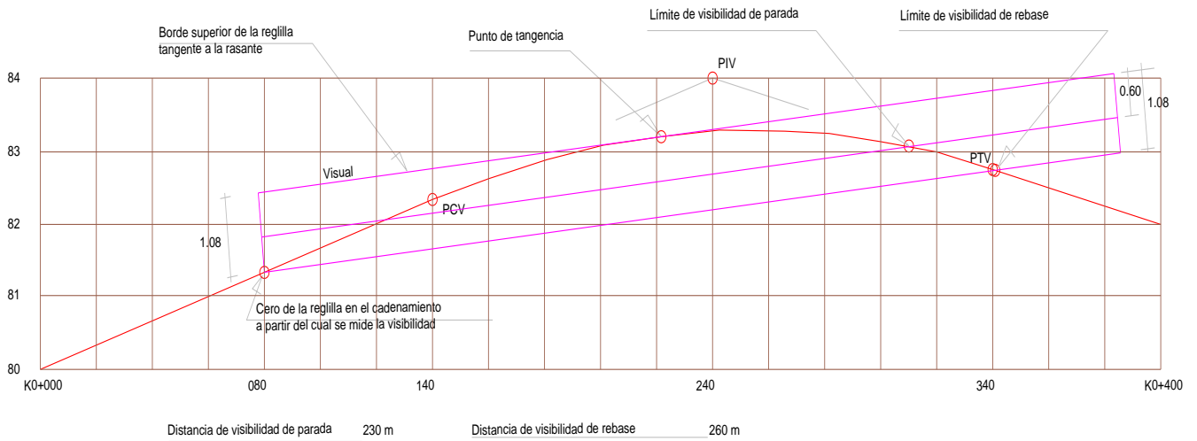
FIGURA I.6. Determinación de distancias de visibilidad en planos.
