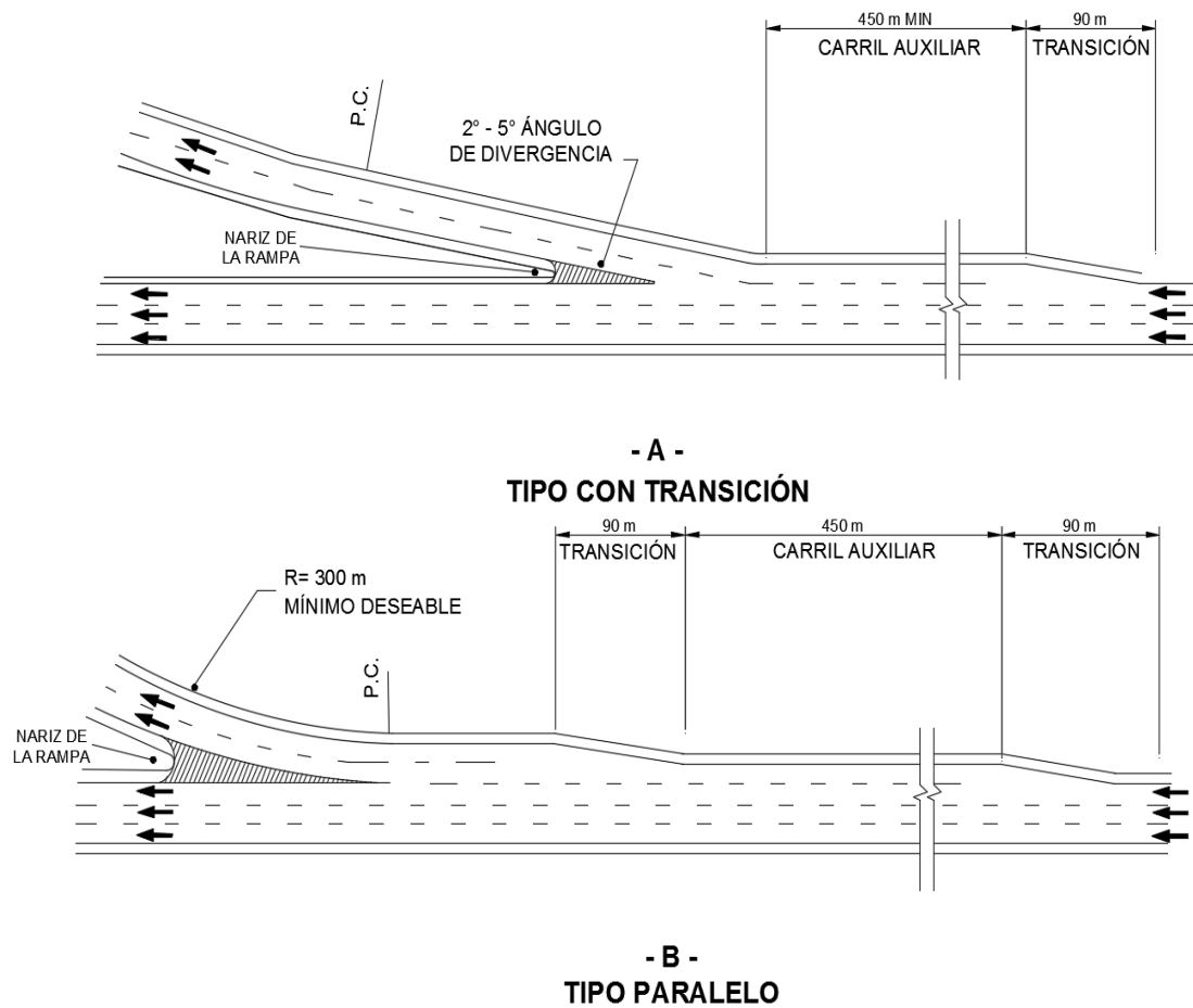
FIGURA VII.48. Extremos de enlaces de salida de dos carriles
