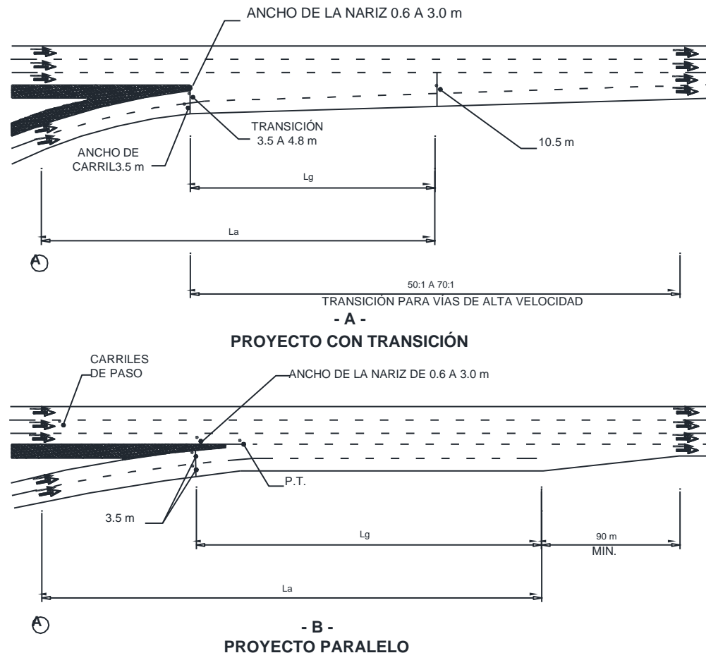
FIGURA IX.37. Enlaces típicos de entrada de dos carriles
