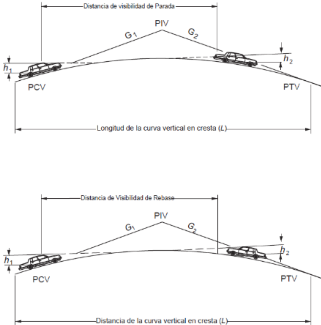
FIGURA III.70.- Parámetros a considerar en la determinación de la longitud de una curva vertical en cresta, para proporcionar la Distancia de Visibilidad de parada
