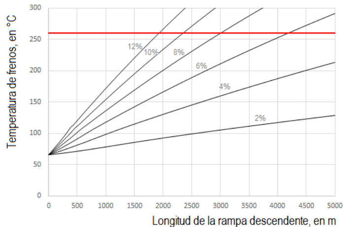
FIGURA II.8. Variación de la temperatura con la longitud las pendientes descendentes
