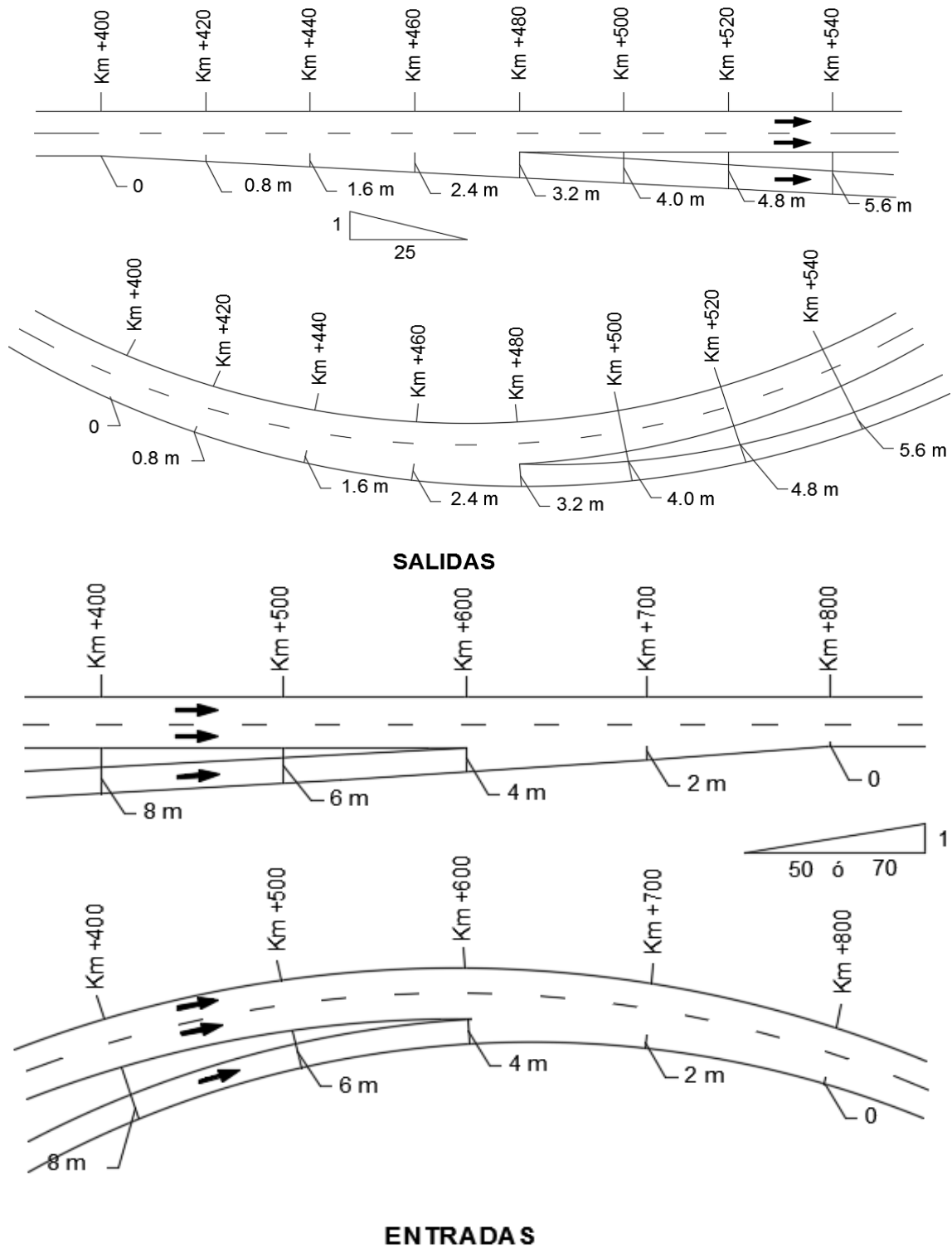
FIGURA. VII.45. Esquema de extremos de enlaces del tipo transición sobre curvas
