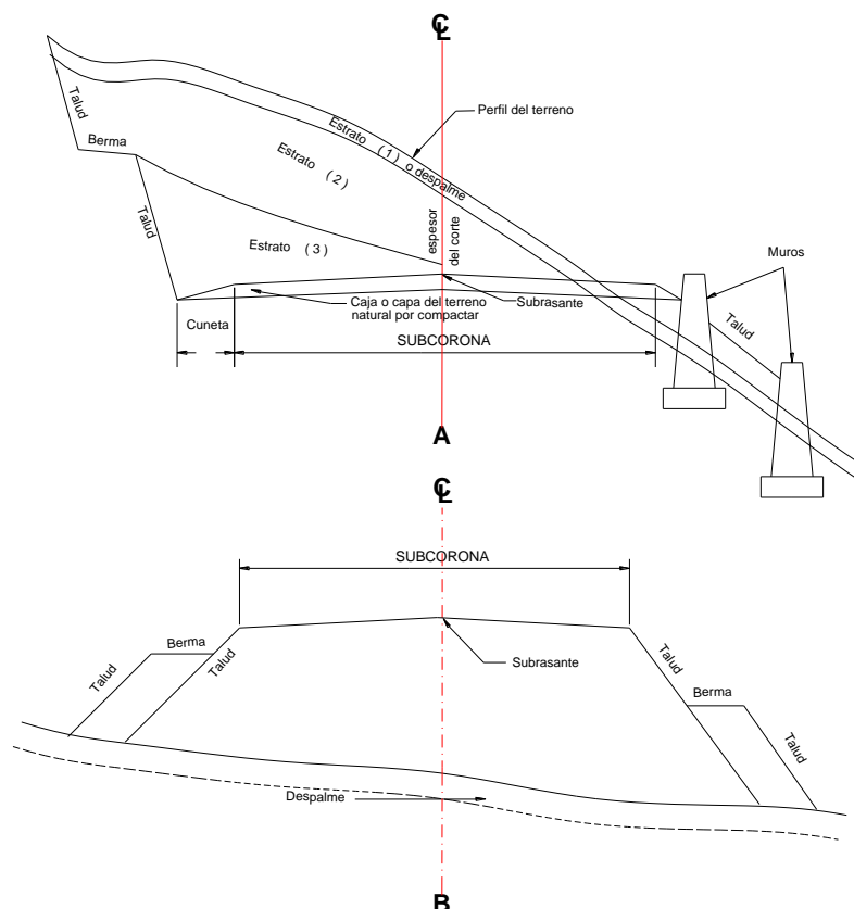
FIGURA VI.4 MUROS Y BERMAS
