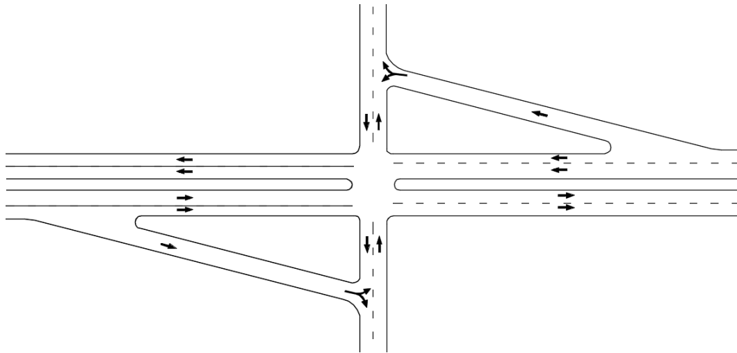
FIGURA VII.27. Intersección con ramales diagonales
