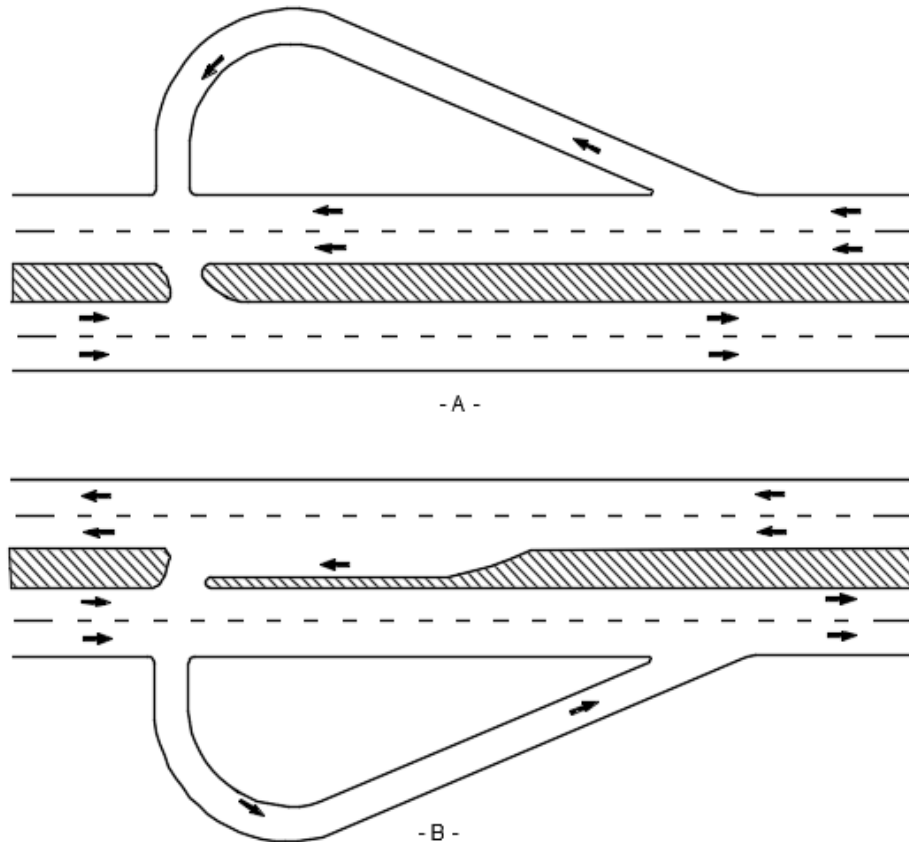
FIGURA VIII.37. Franjas separadoras angostas con carril de vuelta izquierda indirecta
