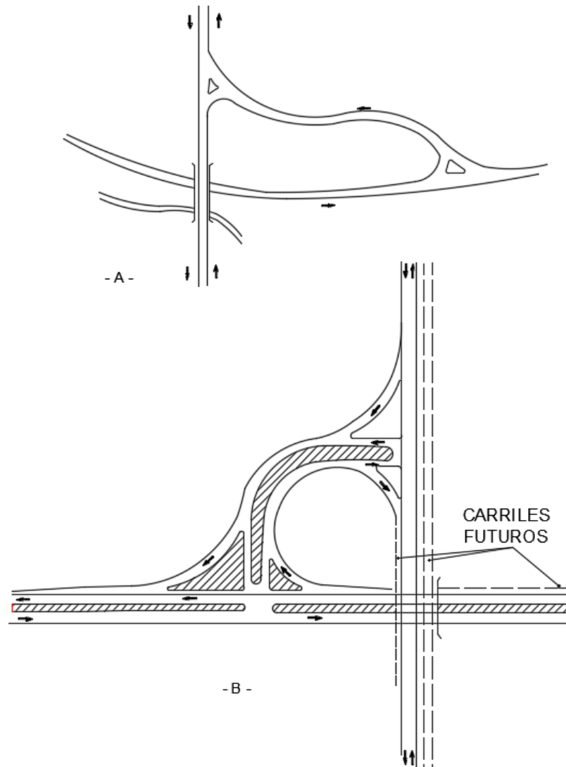
FIGURA IX.7. Intersección de cuatro ramas con enlaces en un cuadrante
