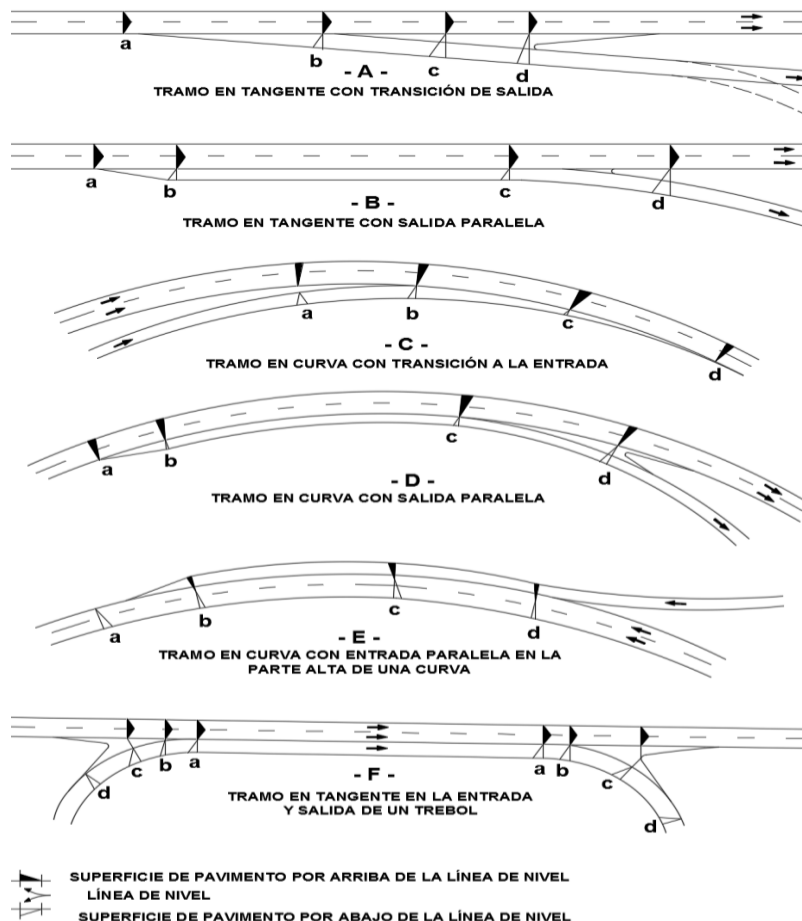
FIGURA IX.29. Desarrollo de la sobreelevación en extremos de enlaces con flujo libre
