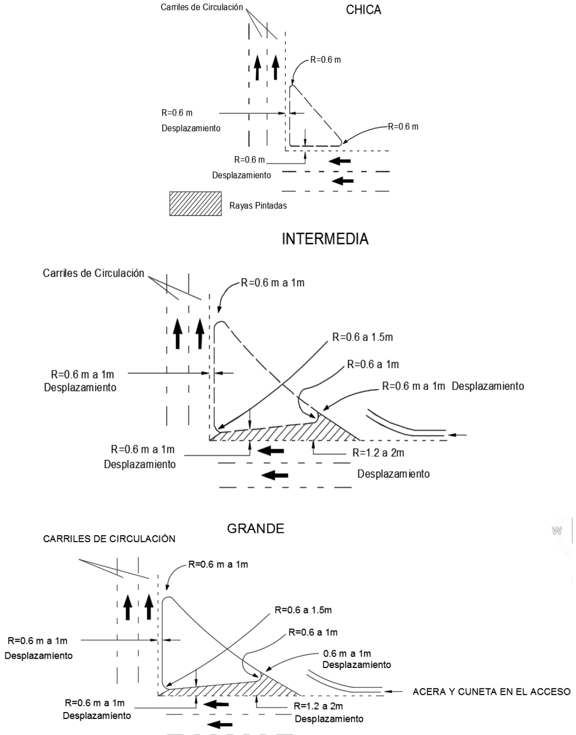
ISLA TRIANGULAR ESQUINADA SOBRE CALLES URBANAS FIGURA VIII.17. Detalles de diferentes proyectos de isletas en esquina para carriles para dar vuelta (ubicación urbana)
