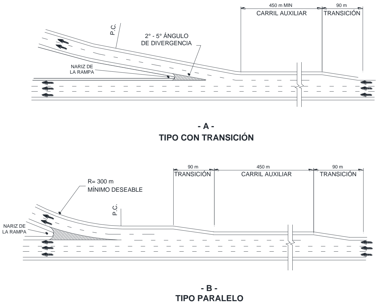
FIGURA IX.38. Extremos de enlaces de salida de dos carriles
