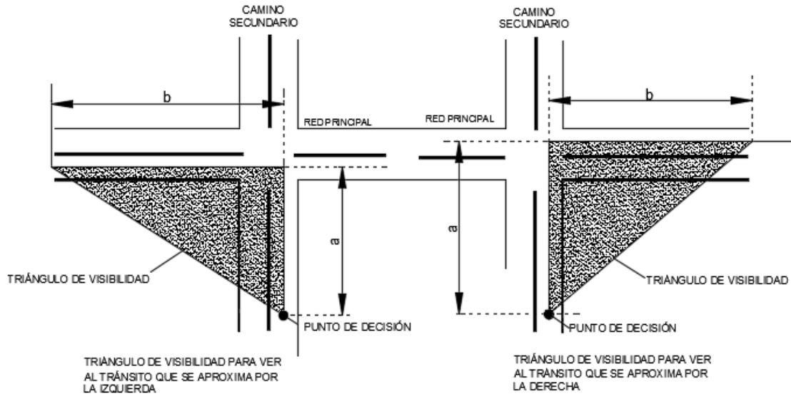
TRIÁNGULOS DE VISIBILIDAD DE LLEGADA
