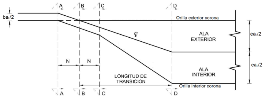
FIGURA II.14. Transición de sobre elevación con giro sobre orilla
