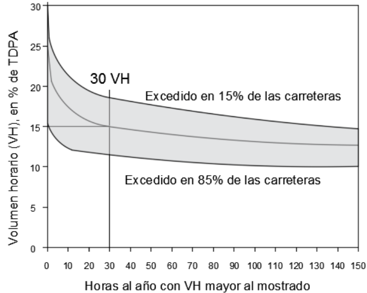
FIGURA I.4. Variación de volúmenes horarios más altos del año
