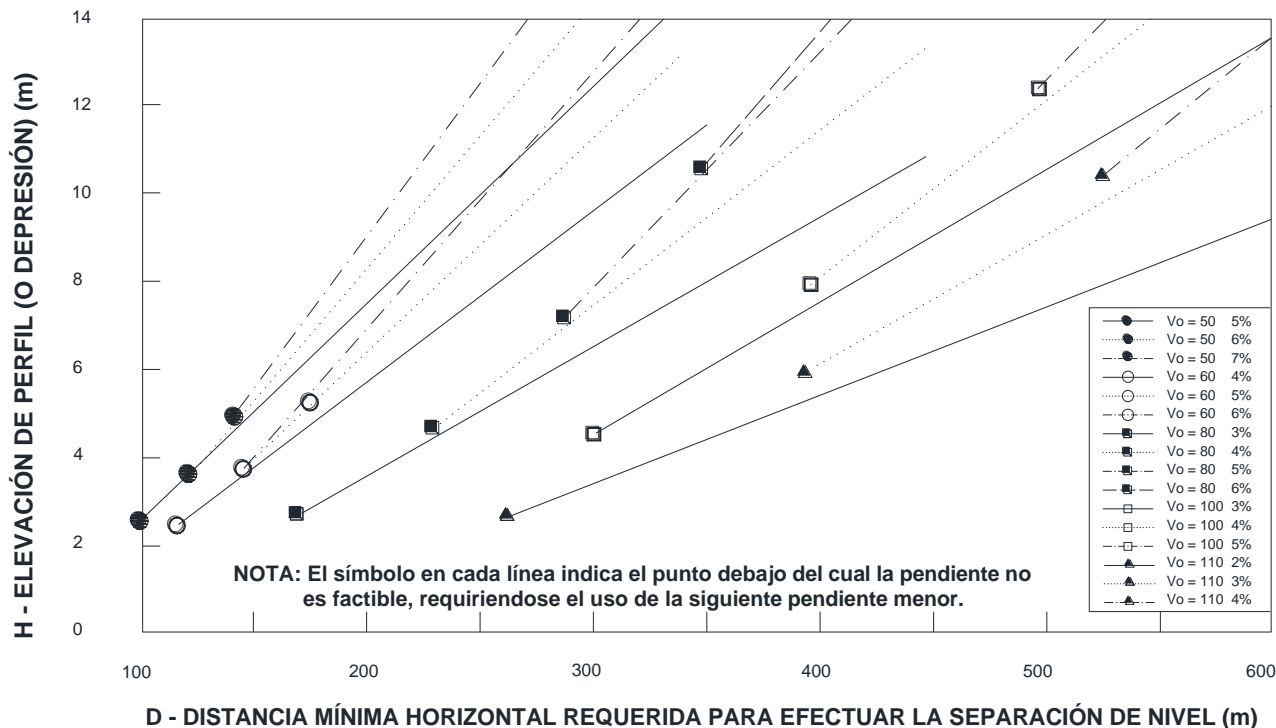
FIGURA IX.44. Terreno plano. distancia longitudinal necesaria para el diseño óptimo de una separación a desnivel
