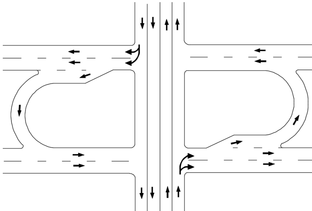
FIGURA VIII.35. Vueltas izquierdas indirectas alrededor del entronque
