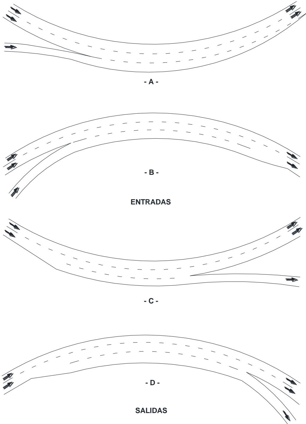
FIGURA IX.36. Extremos de enlaces de tipo paralelo sobre curvas
