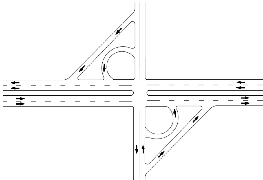
FIGURA VII.28. Intersección con ramales tipo medio trébol
