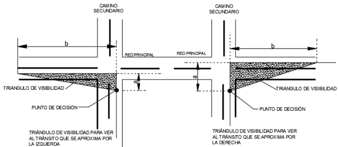
TRIÁNGULOS DE VISIBILIDAD DE SALIDA
