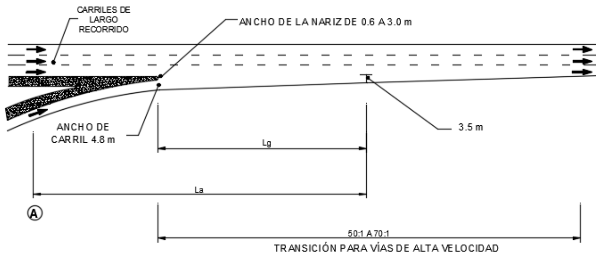
- A - PROYECTO CON TRANSICIÓN
