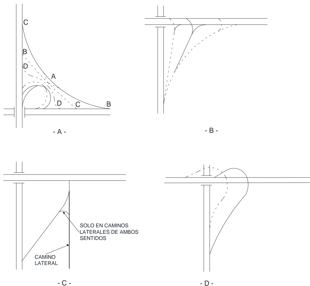
FIGURA IX.28. Formas de enlaces
