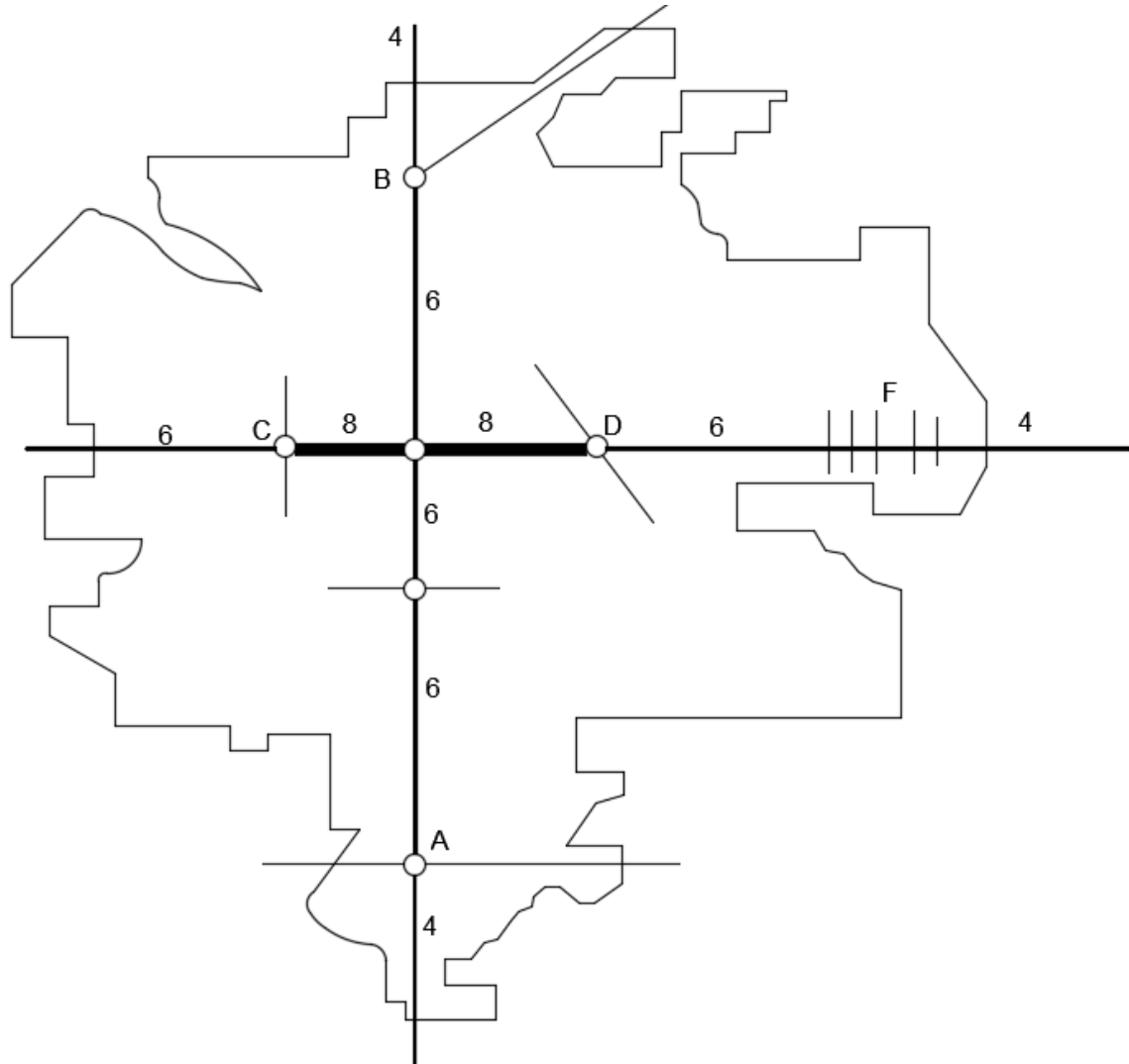
FIGURA IX.20. Representación esquemática del número básico de carriles
