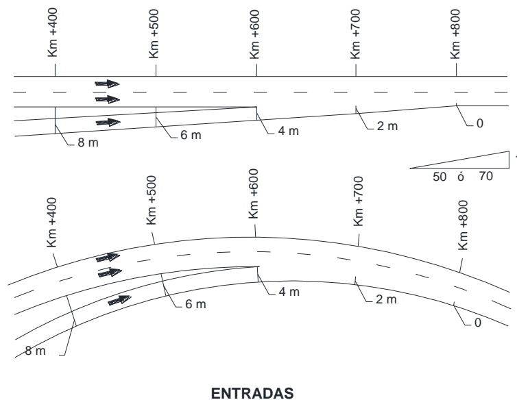
FIGURA IX.35. Esquema de extremos de enlaces del tipo transición sobre curvas
