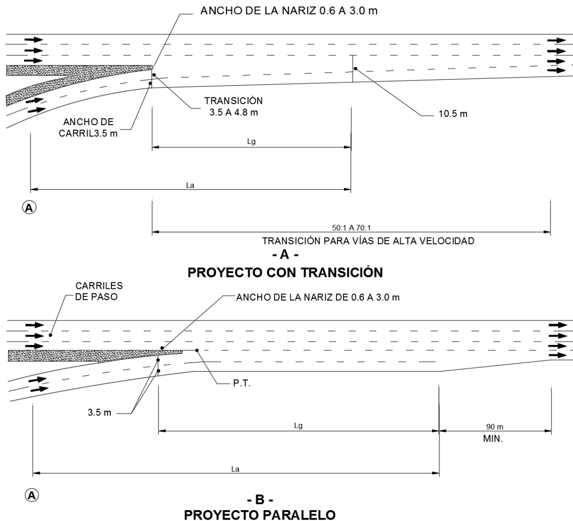
FIGURA VII.47. Enlaces típicas de entrada de dos carriles
